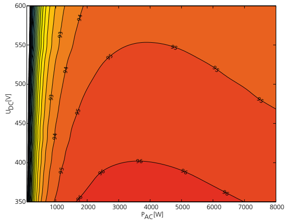
3D-Wirkungsgraddiagramm Powador 9600
